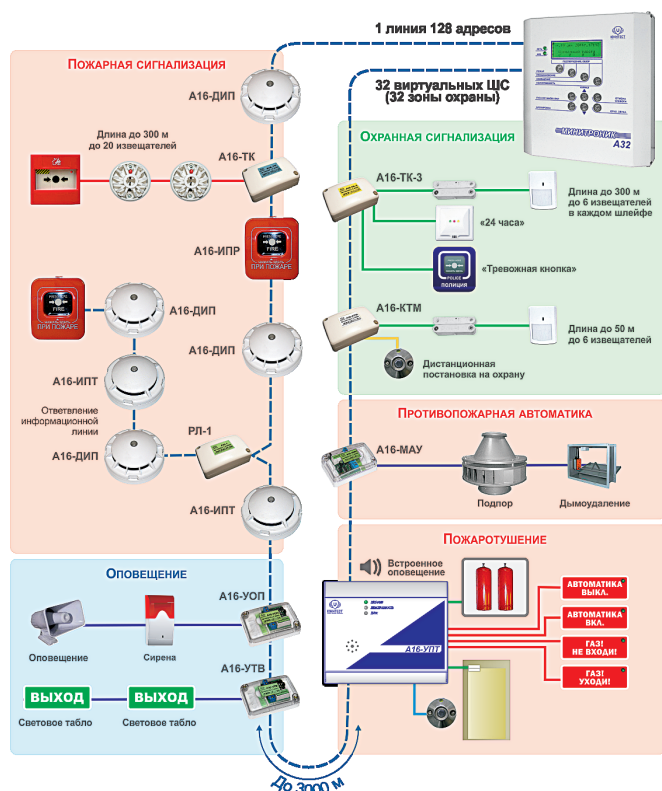
Структурная схема подключения устройств
