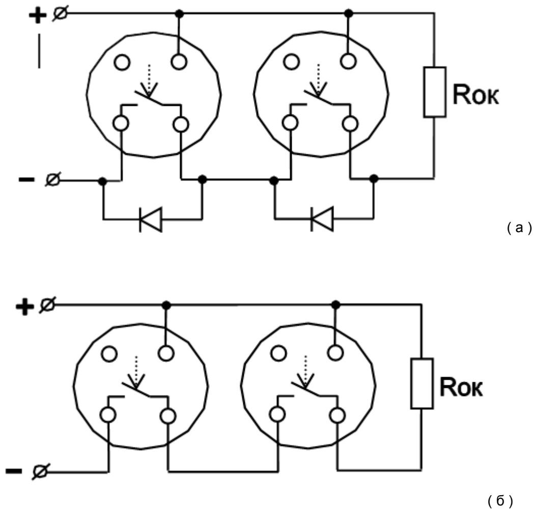
Рис.1. Схема включения извещателя «с подтверждением исправности»: а – в знакопеременный шлейф сигнализации (диод включен в состав извещателя); б – в однополярный шлейф сигнализации.
