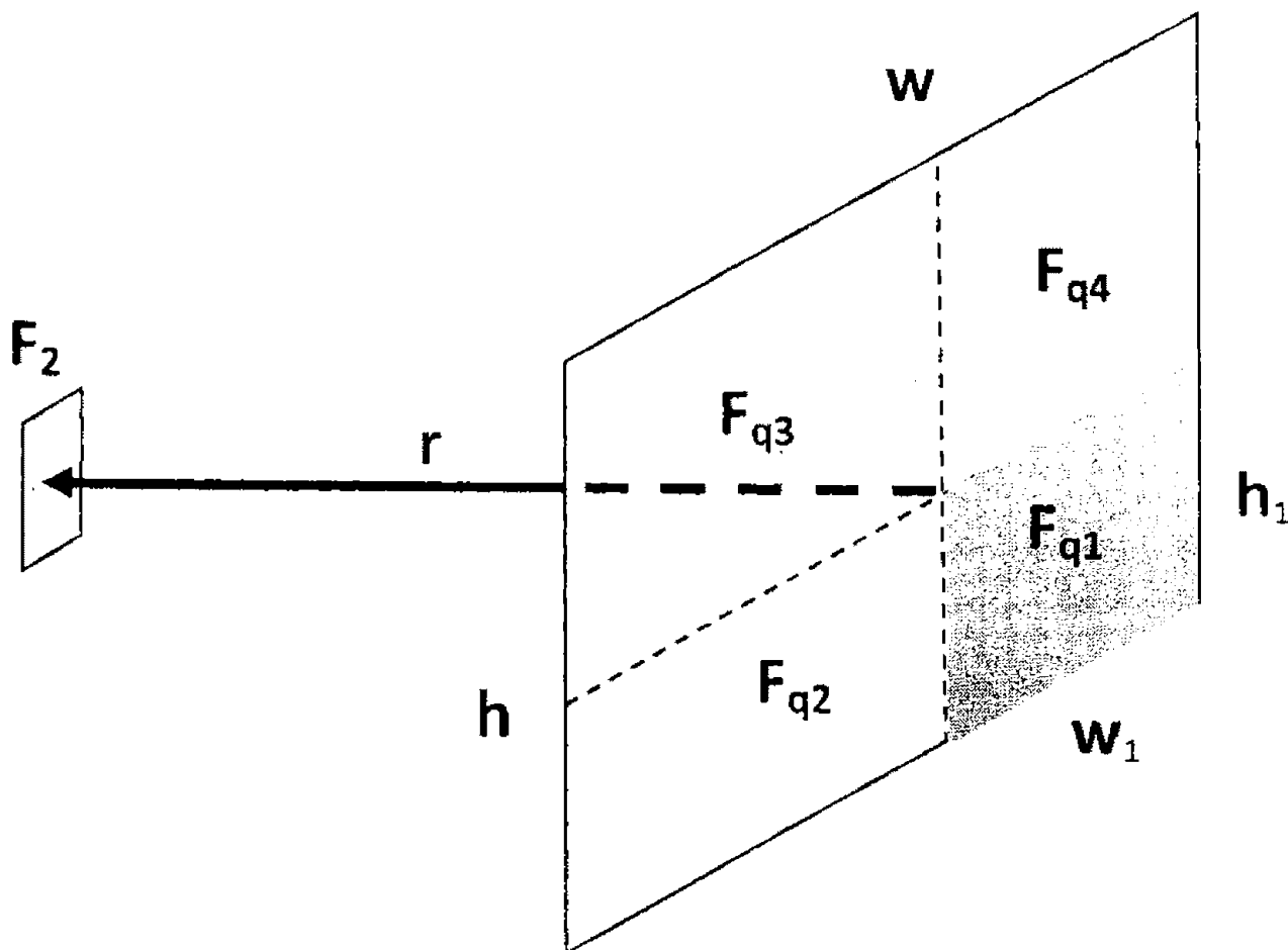
Рисунок А.3.2. Расположение излучающих поверхностей пламени
