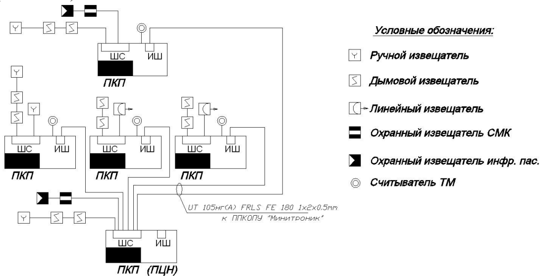
Рис.4. Схема объединения ПКП «Минитроник» в древовидную сеть с помощью шлейфов сигнализации (ШС) и имитатора шлейфа (ИШ).
