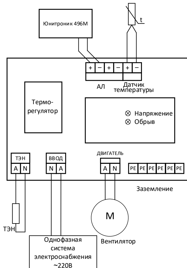
Рис.5. Схема подключения ШУП-3 исп.1К220/220.
